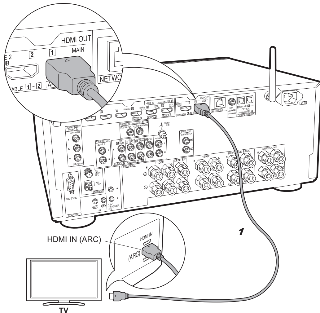
1 HDMI cable
