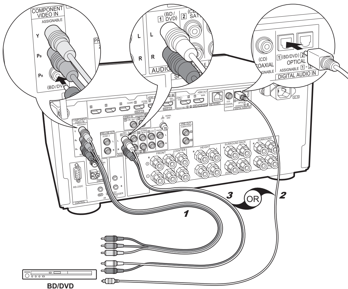
1 Câble vidéo composante, 2 Câble optonumérique, 3 Câble audio analogique
