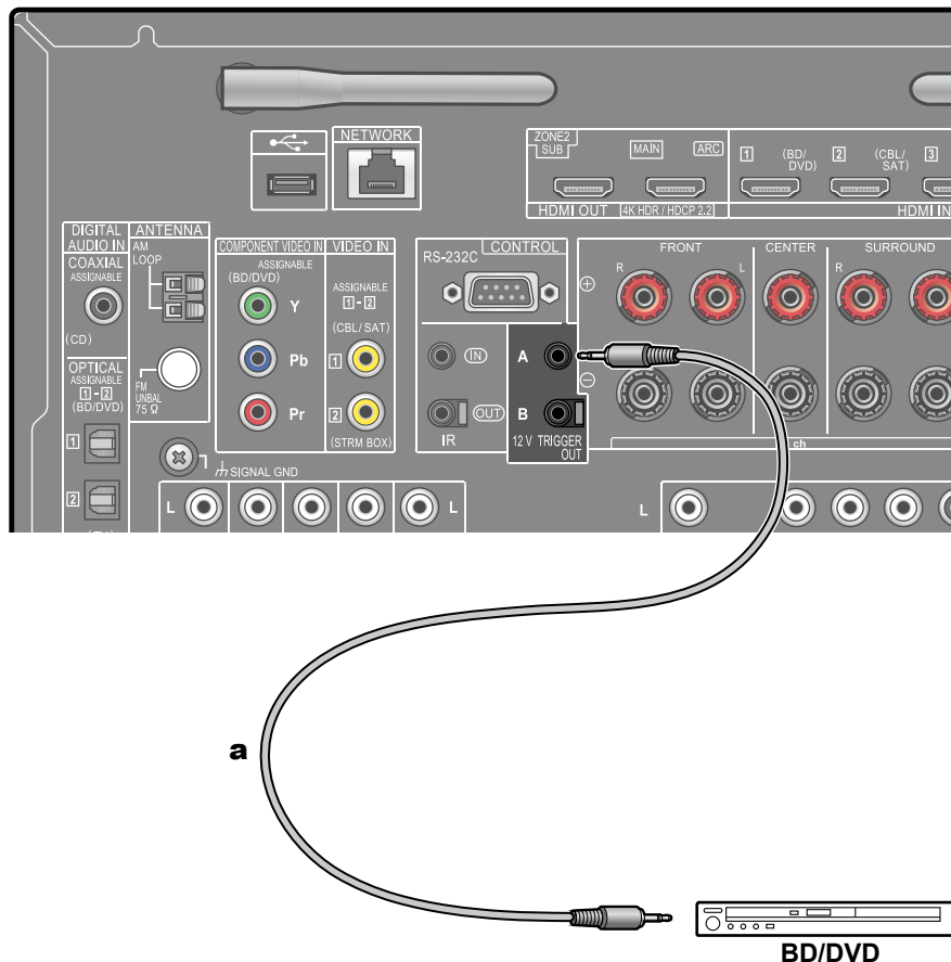
a Monaural mini plug cable (ø1/8"/3.5 mm)
