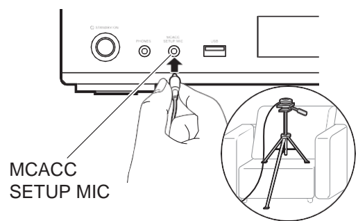
Пример установки микрофона настройки АС см. на рисунке.
