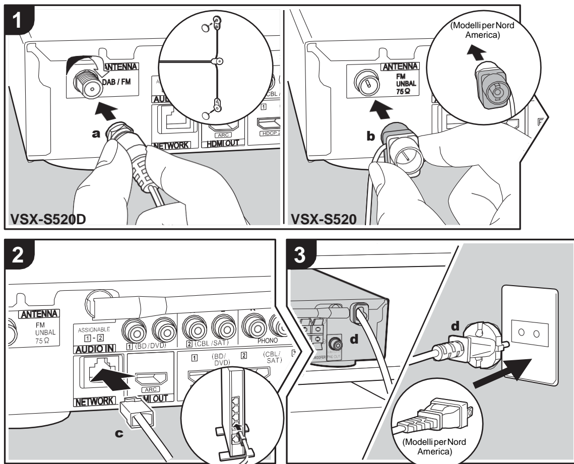
a Antenna DAB/FM, b Antenna FM per interni, c Cavo Ethernet, d Cavo di alimentazione
