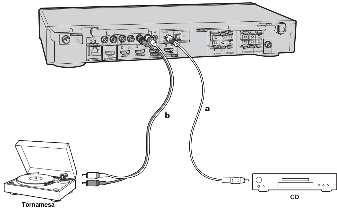
a cable coaxial digital, b cable de audio analógico
