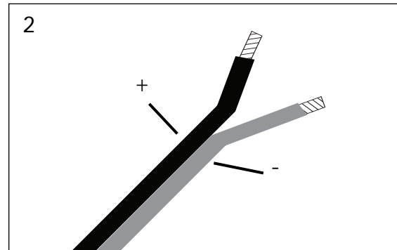
Identify markings on wire and assign +/-. Identifique las marcas de positivo (+) y negativo (-). Identifiez les repères sur le câble et respectez les polarités +/-.
